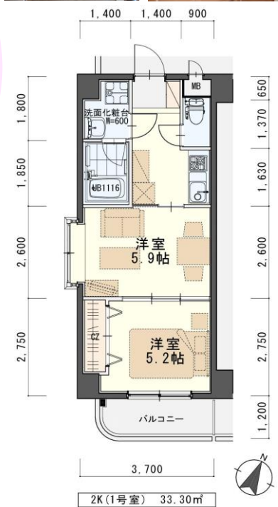
2K(1号室) 33.30㎡
